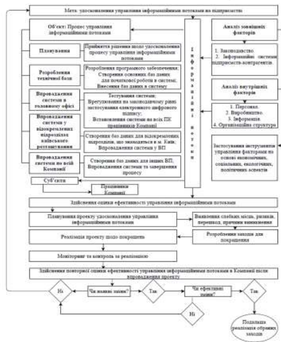
Алгоритмічна модель
